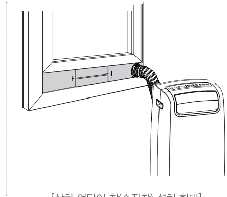
[상하 여닫이 창(수직창) 설치 형태]
